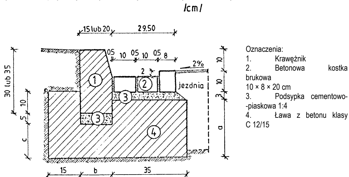
Wymiary uzupełniające (a, b, c)
