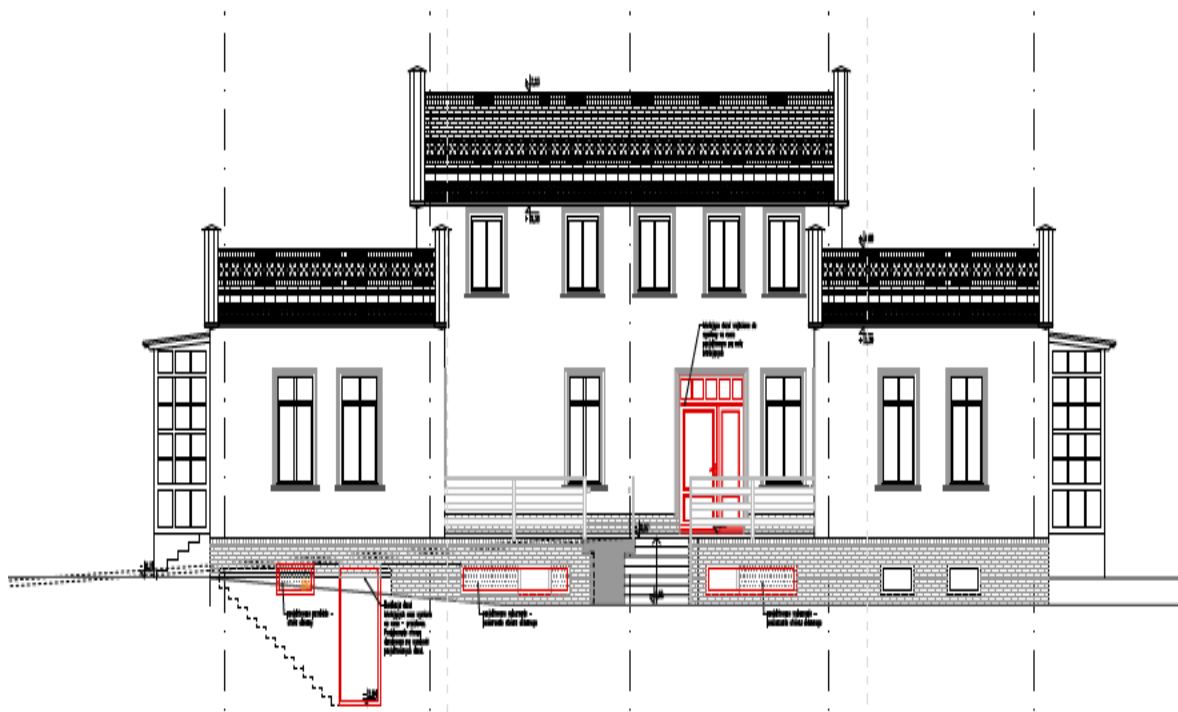
Rysunek 36 Wstępna koncepcja COA
